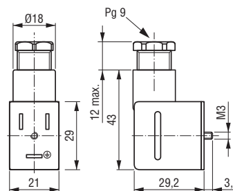
Conector Retangular DIN 43650 forma B
