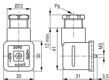
Conector Quadrado DIN 43650 forma A
